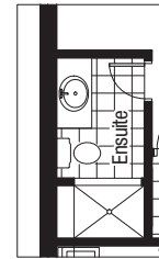
Ensuite Plan Opt. Layout
